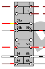
Klemmleiste B
